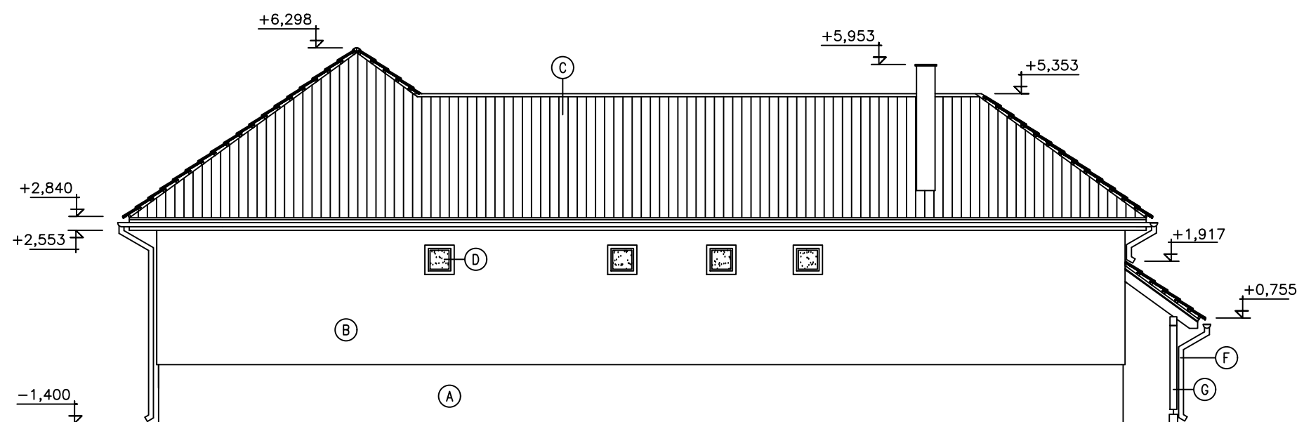
SEVEROZÁPADNÝ POHĽAD
