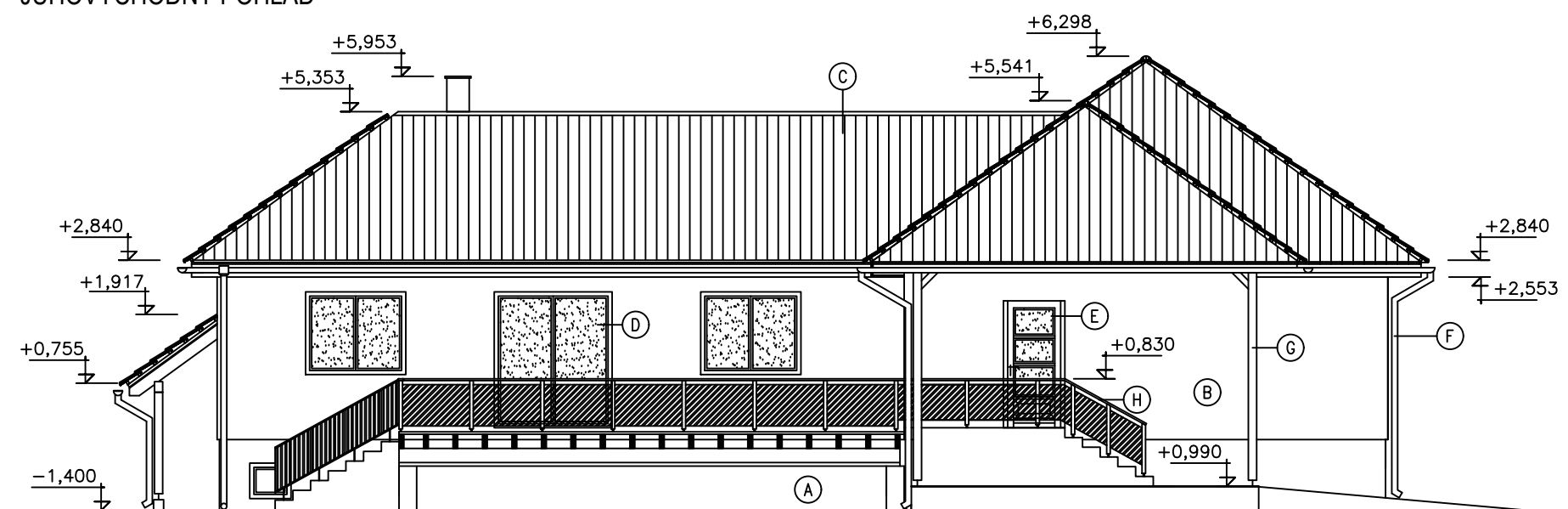
JUHOVÝCHODNÝ POHĽAD
